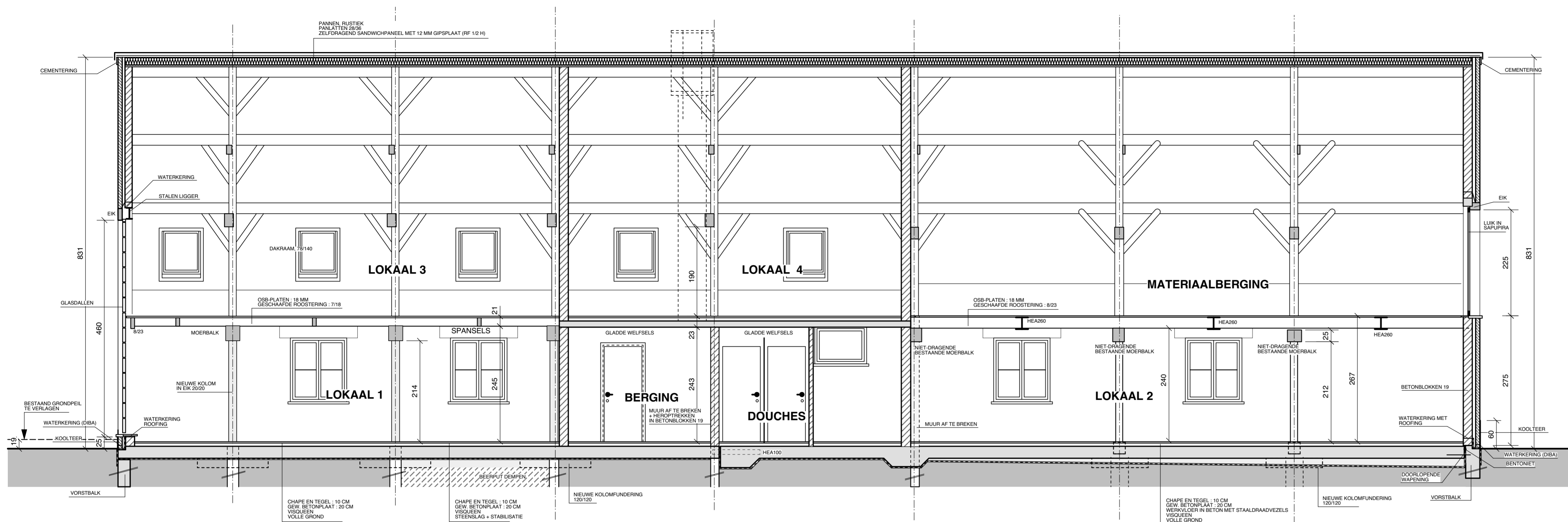
DOORSNEDE AA ontwerp
